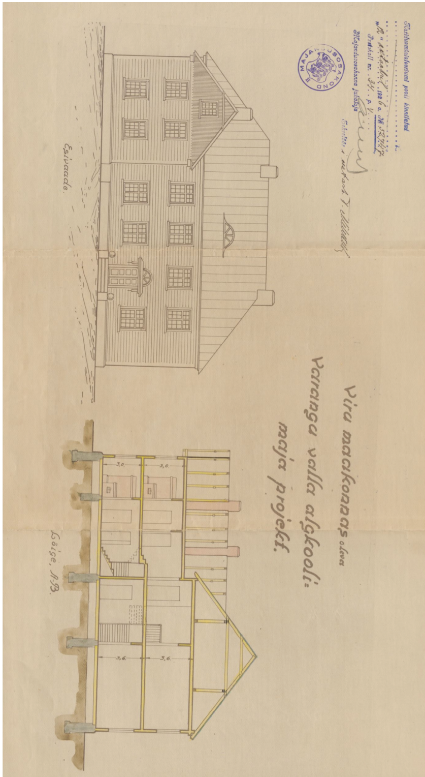
Lisa 1. Hoone algne projekt.
