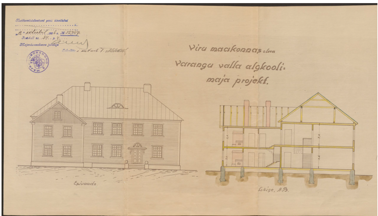
Illustratsioon 1.1. Varangu valla algkooli maja projekt. Vaade peafassaadile ja lõige.
