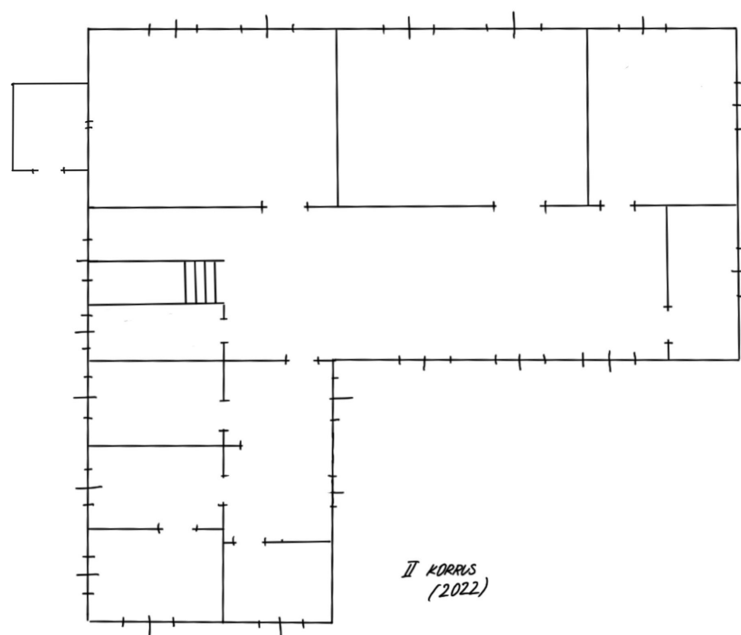
Illustratsioon 1.7. Hoone II korruse põhiplaan 2022. aastal. Plaani koostanud autor.
