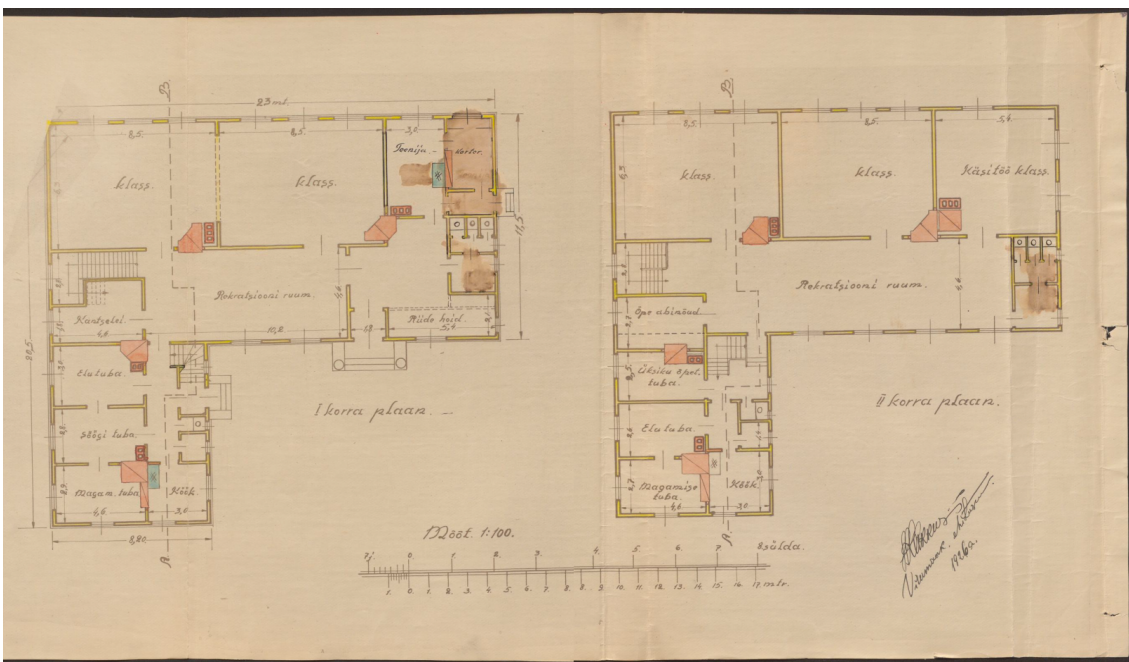
Illustratsioon 1.3. I ja II korruse põhiplaan 1930 a.
