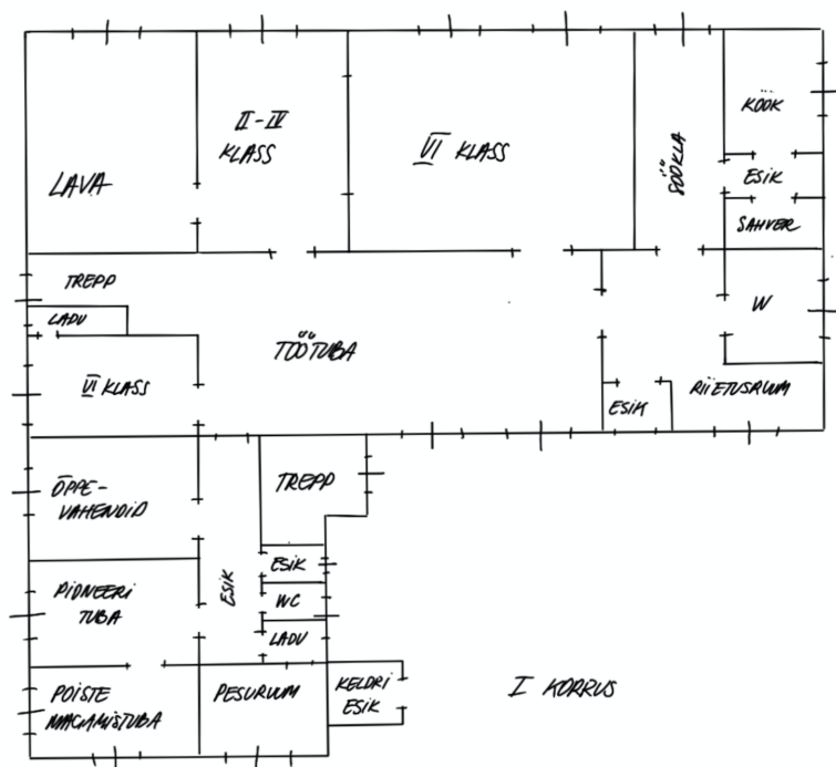
Illustratsioon 1.4. Maja plaan, koostatud 1956. aastal, 1. korrus. Eskiiside põhjal koostanud autor.
