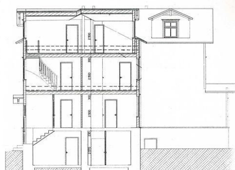
Maja 1 lõige
