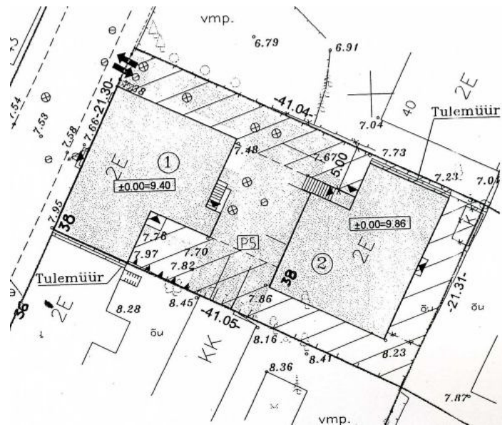
Asendiplaan
