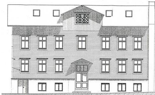
Maja 1 eestvaade
