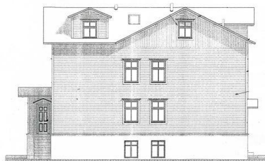
Maja 1 otsavaade
