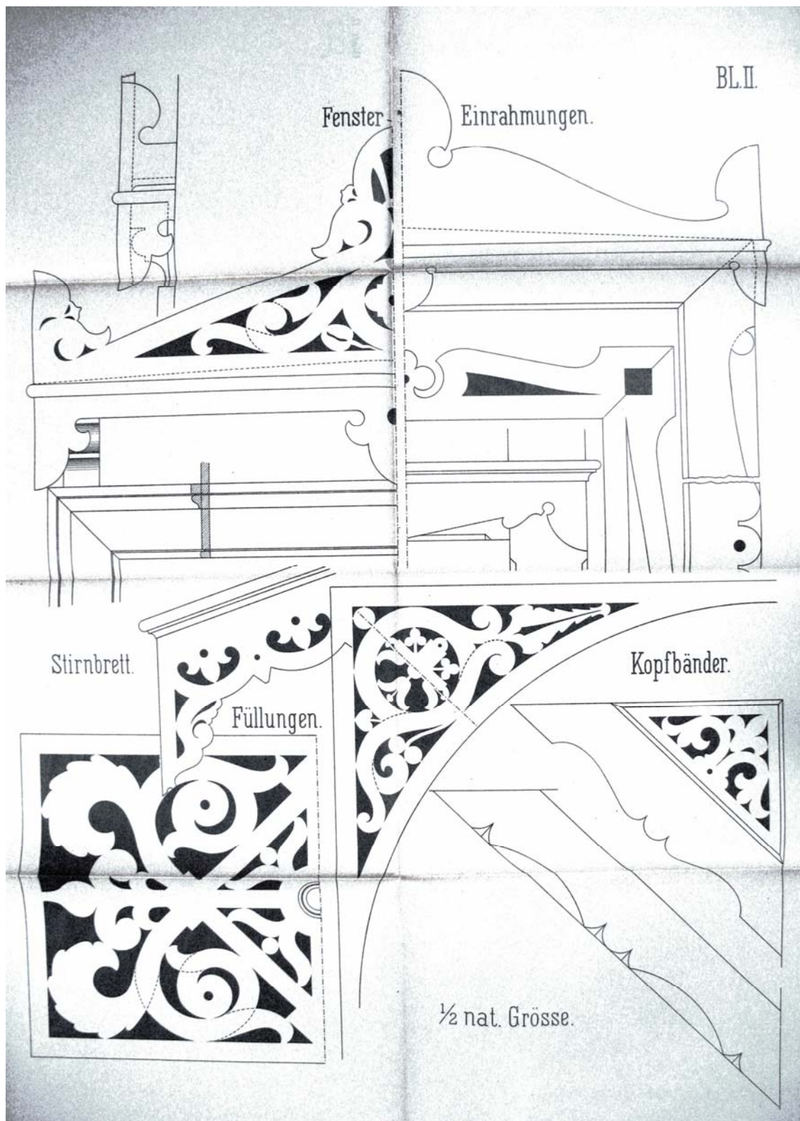
2.) Puitdekoori elemendid (leht II)
