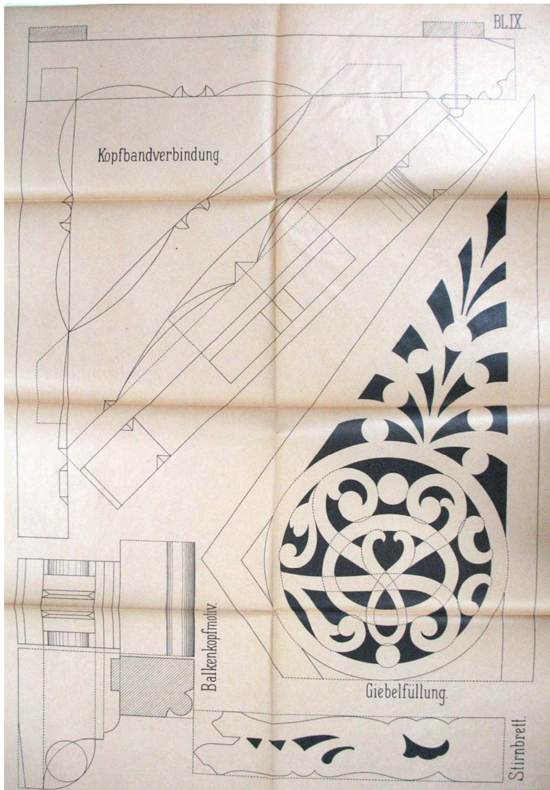
9.) Puitdekoori elemendid (leht IX)
