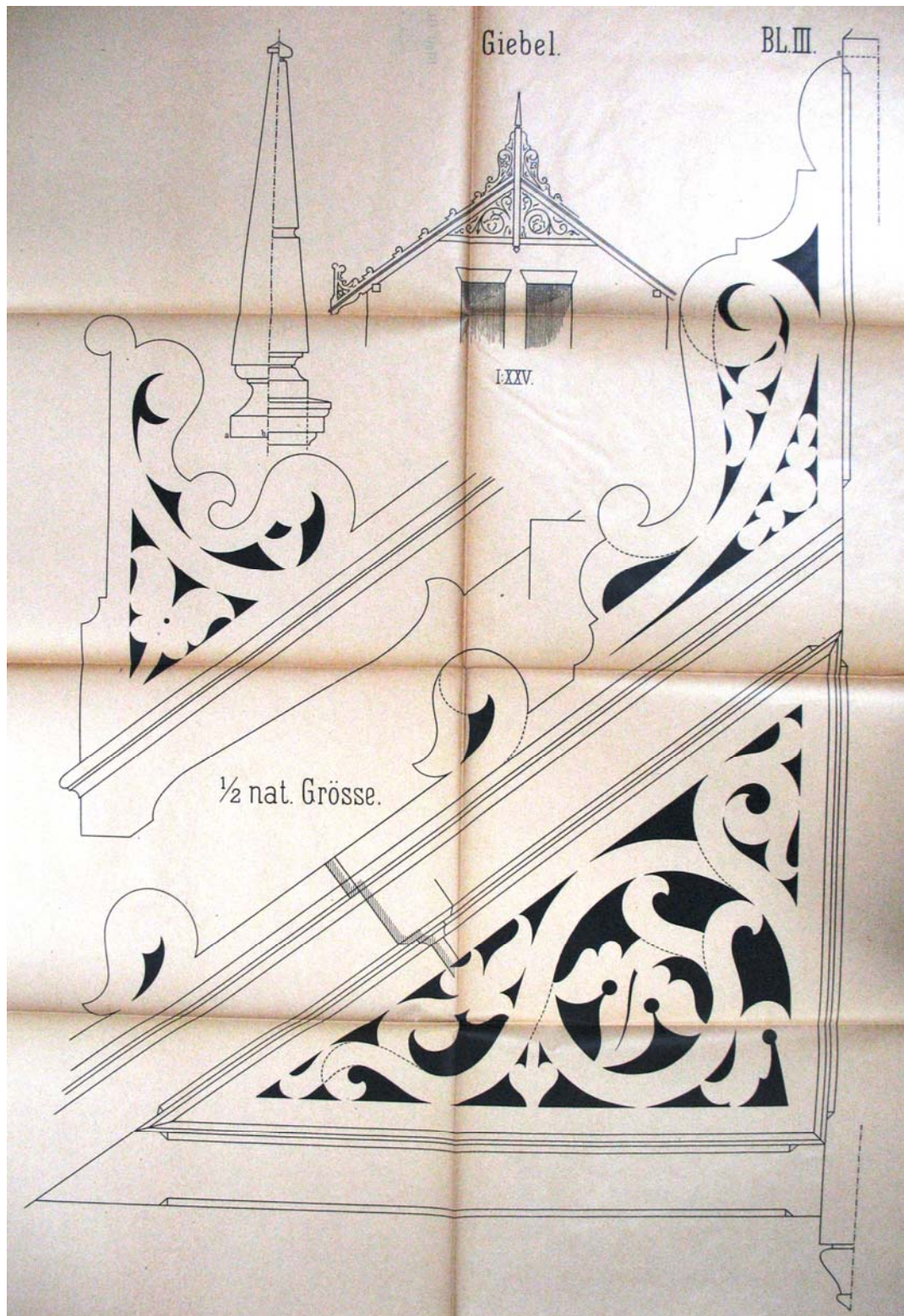
3.) Puitdekoori elemendid (leht III)
