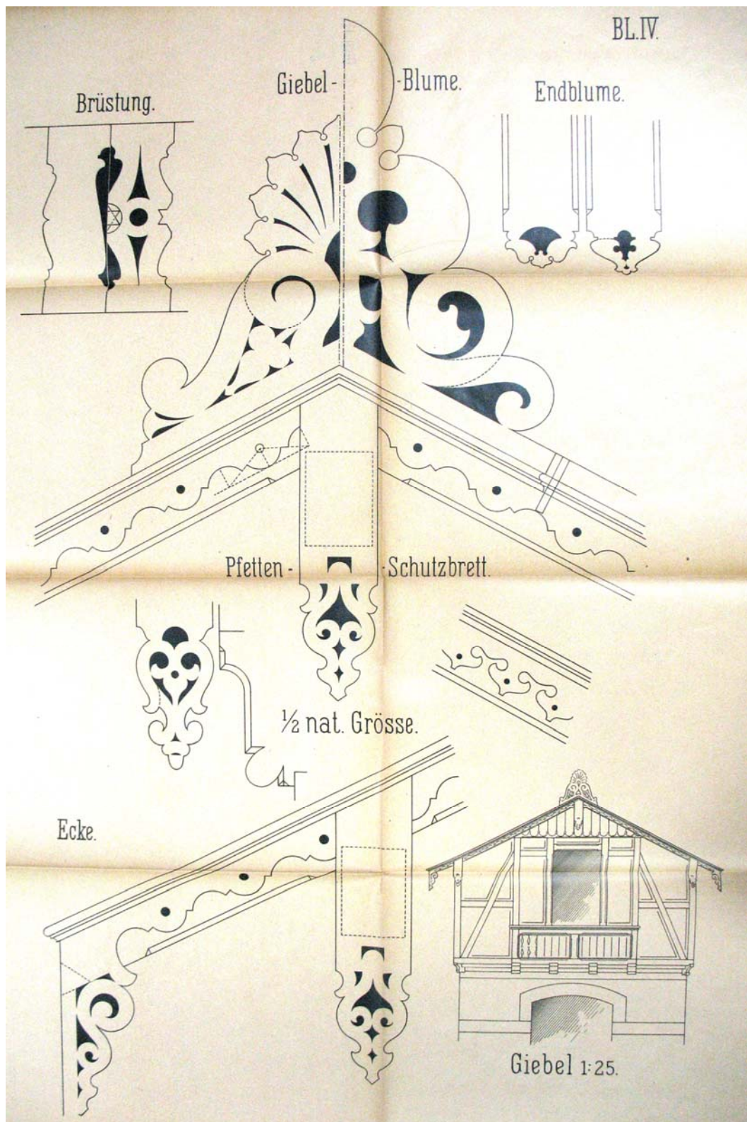
4.) Puitdekoori elemendid (leht IV)
