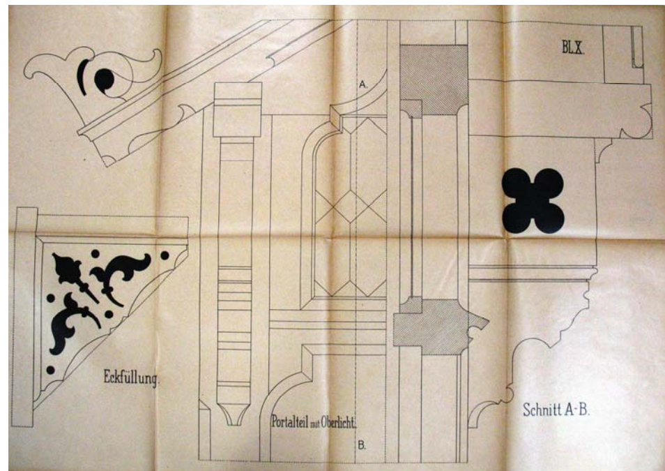
10.) Puitdekoori elemendid (leht X)
