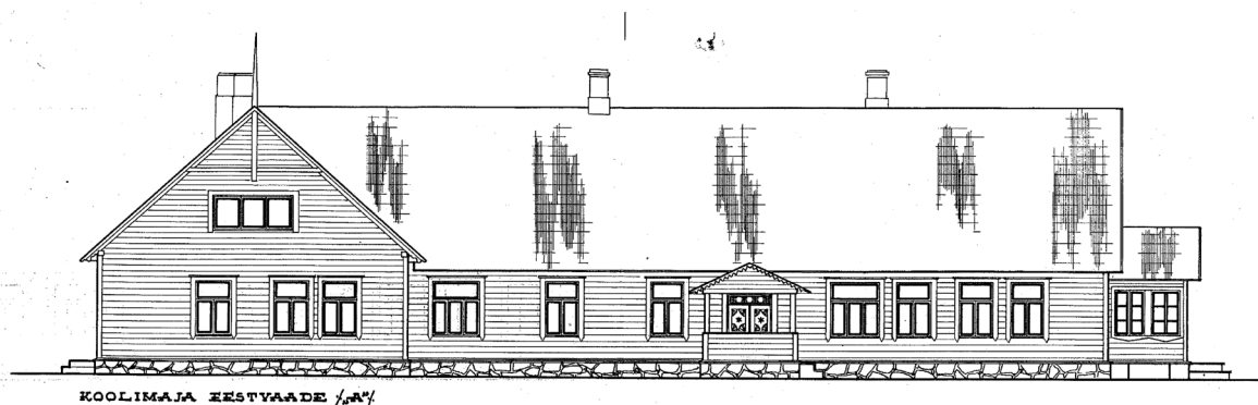
KOOLIMAJA EESTVAADE 1/2002
