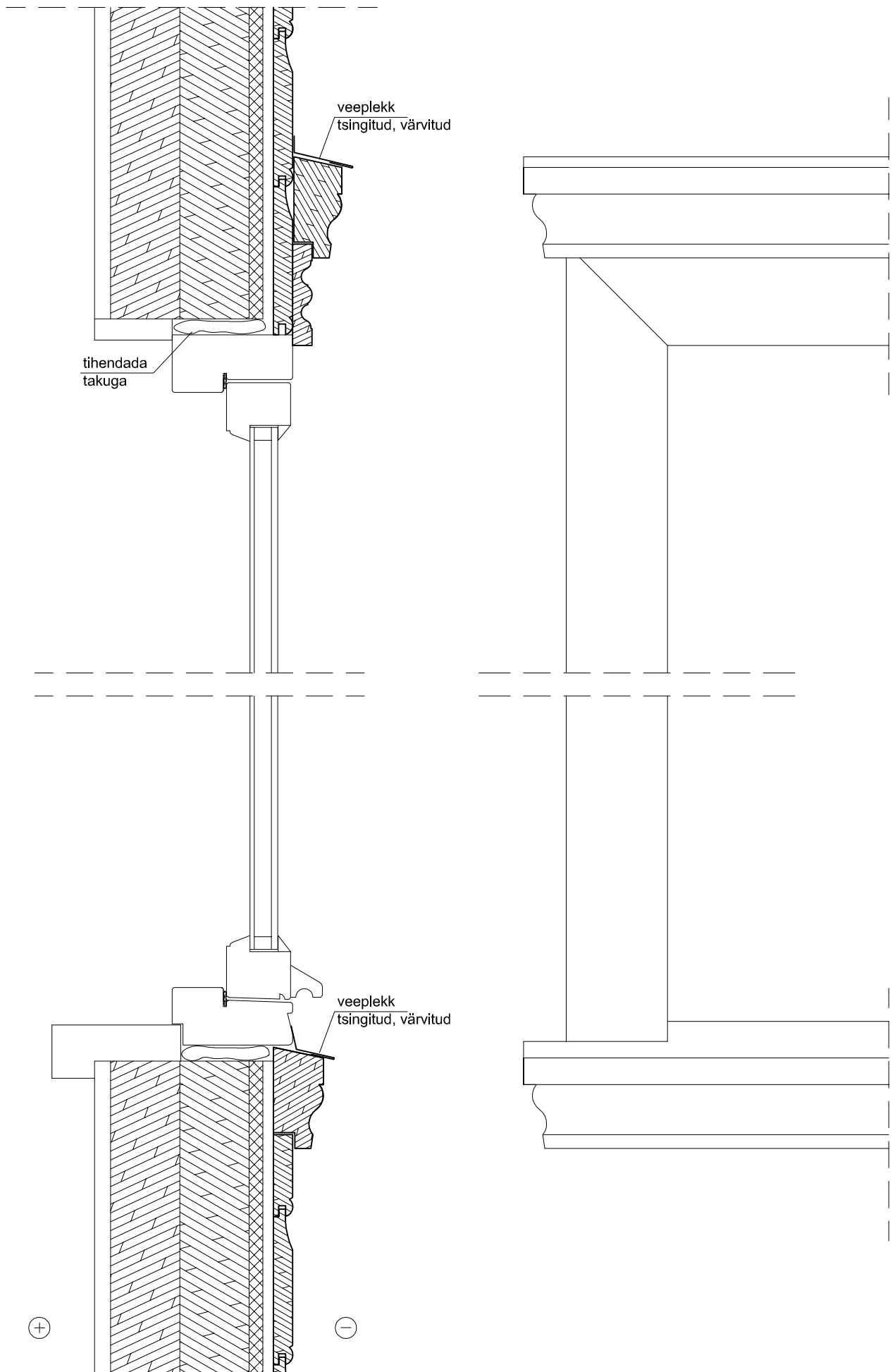
AKNA ÜMBRISLAUAD VERTIKAALNE LÕIGE JA VAADE
