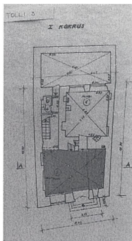
Lae asukoht hoone põhiplaanil
