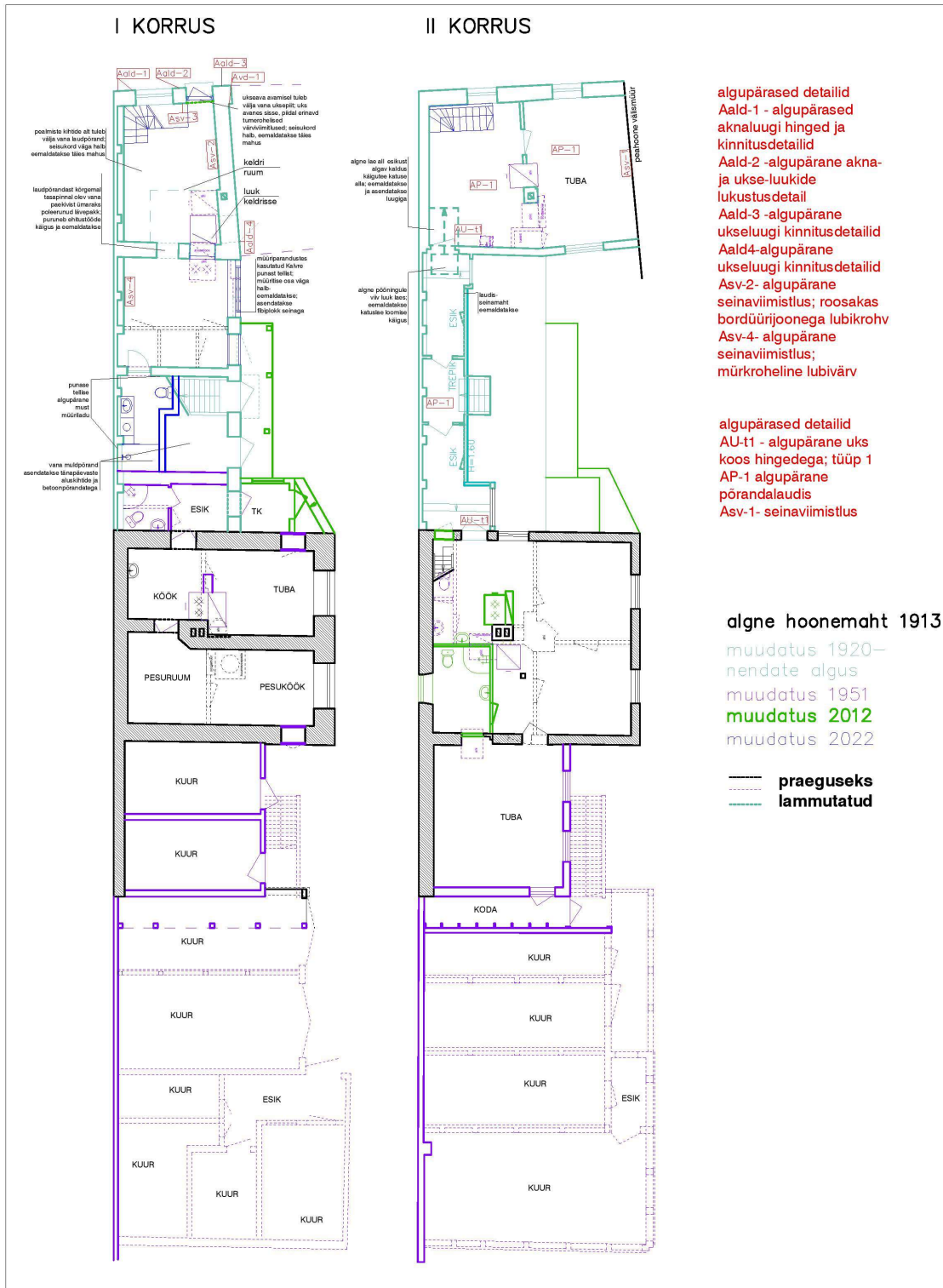
Joonise autor; Liis Tarbe 2023 aastal Joonised koostatud Agnes Joala 2019 aastal teostatud mõõdistusjooniste põhjal
