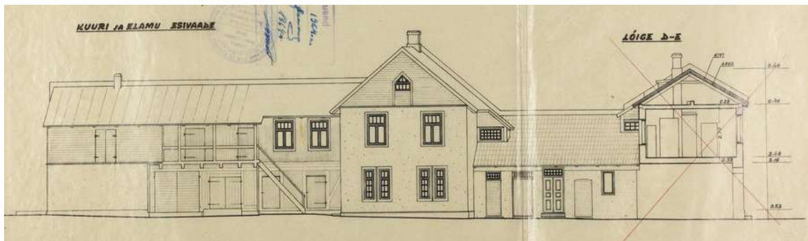
Joonisel näha praeguseks lammutatud kuuride maht ja praeguseks oluliselt teisenenud akendejaotus
