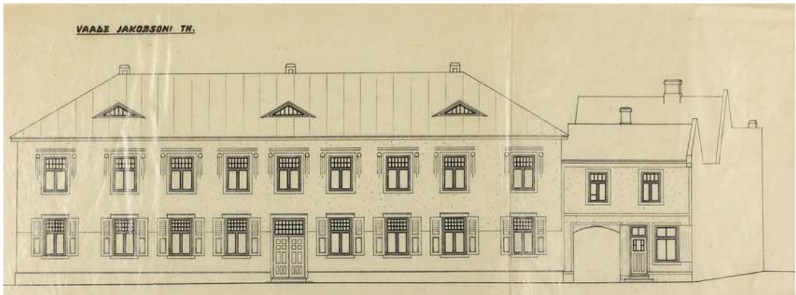
Joonisel on alla kirjutatud, et tegu on looduses ülesse mõõdetud hoone plaanide/joonistega. Fassaadil näha olev juugend-dekoor ei ole „mäletavte elanike“ sõnutsi kunagi teostunud, küll on tõene akende raamistiku jaotised. Peamaja krohvi uuendamisel võiks siiski teha varasemate krohvikihide uuringu.
